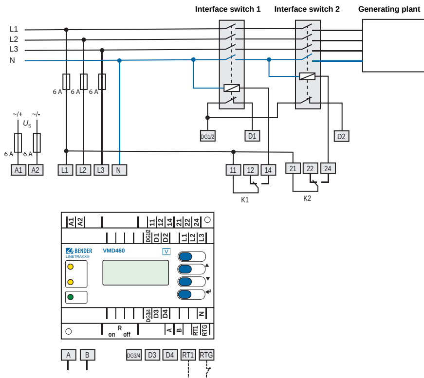
Fig. 4.5: Esquema de conexiones VMD460-NA (programas básicos G98, G99, C10/11, 0126)
