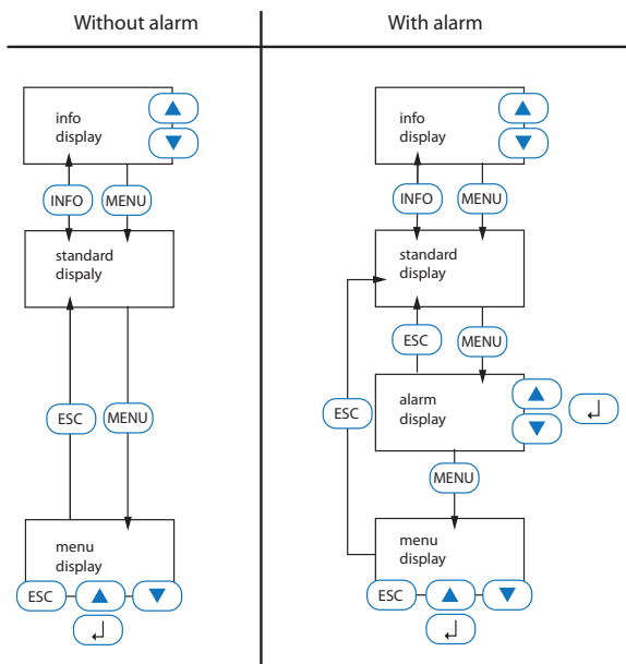
Fig. 5.5: Cambio entre las diferentes pantallas (con o sin alarma)
