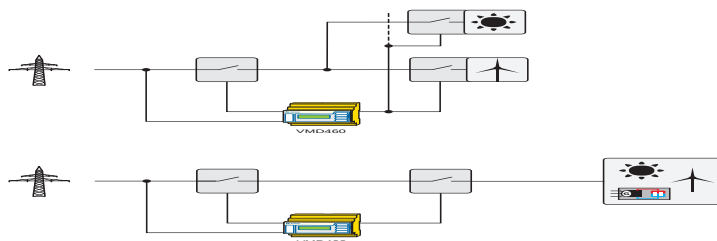
Fig. 4.1: Esquema de conexiones de una protección central RI con interruptores del sistema según VDE-AR-N 4105:2018-11
