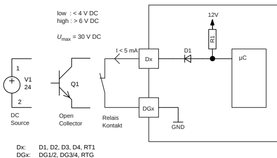
Fig. 4.7: Diagrama de bloque (representación simplificada)
