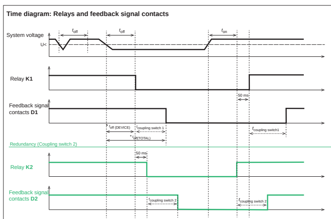
Fig. 7.1: Comentarios sobre el diagrama de tiempos de actuación:
