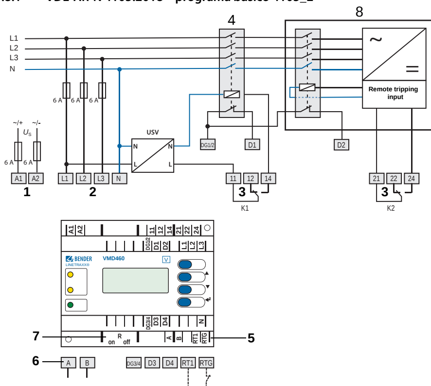
Fig. 4.3: Esquema de conexiones VMD460-NA - programa básico 4105_2
