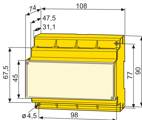
Fig. 4.2: Diagrama de conexiones y plano para fijación por tornillos
