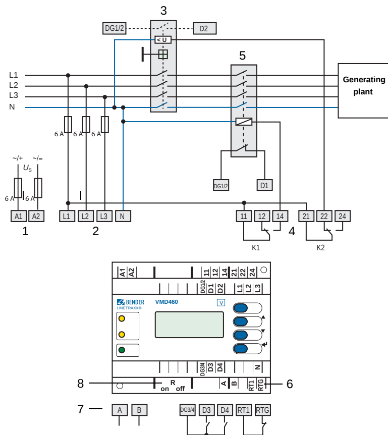
Fig. 4.6: Esquema de conexiones VMD460-NA (CEI 0-21)
