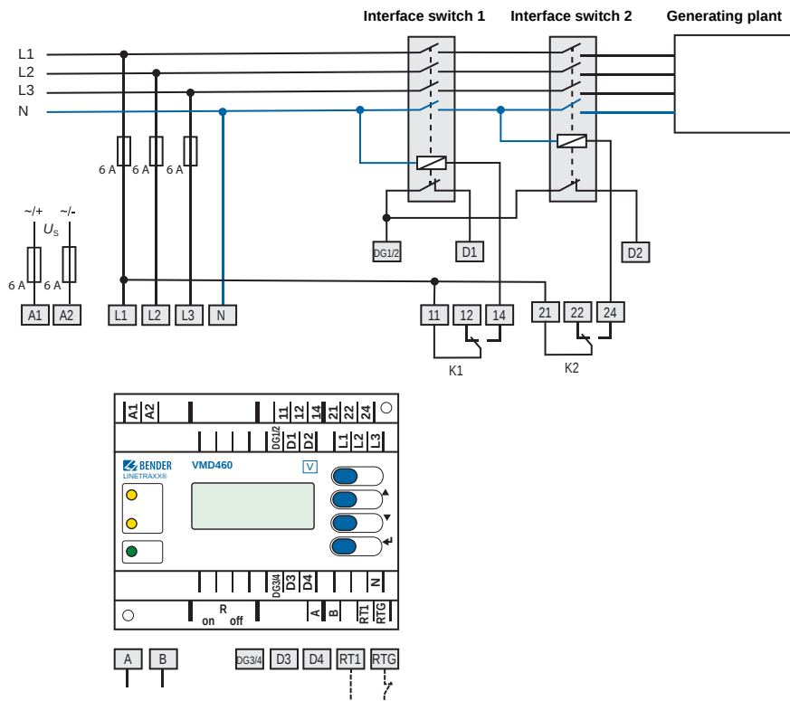
Fig. 4.8: Esquema de conexiones VMD460-NA (programa básico 4105_1, BDEW, G59/3, G83/2)
