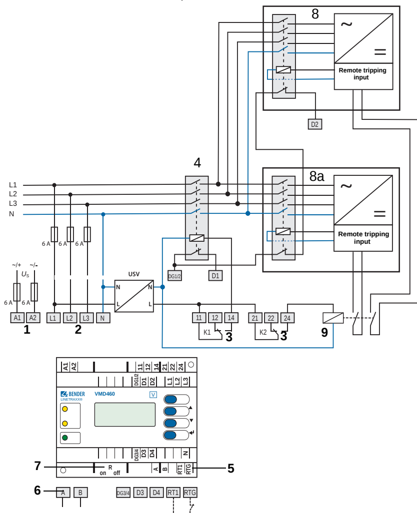
Fig. 4.4: Esquema de conexiones VMD460-NA - Programa básico 4105_2 con varias unidades de generación
